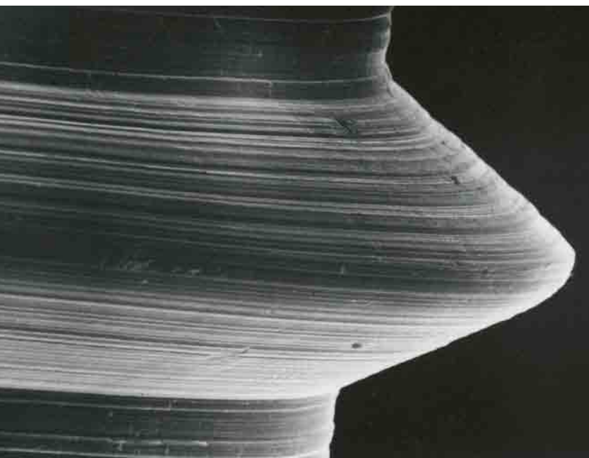
Figur IV. Vårt första implantat var maskinbearbetat, svarvat, och svarvspåren är lätt synliga på denna minimalt råa implantatyta.
